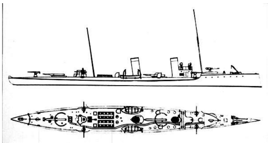
Vista laterale e piano di coperta
